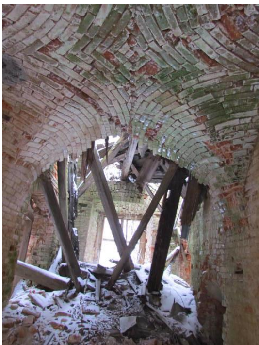
Jediná zaklenutá místnost prvního patra (pravděpodobně modlitebna) v severovýchodním křídle před a po odstranění dřevěných konstrukcí.
