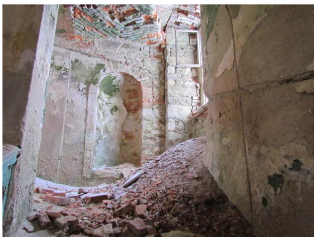
Stav hlavního schodiště před sanací a po vyklizení sutě
